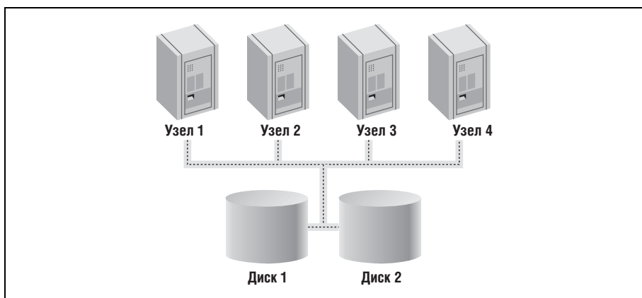
Рис. 9.6. Архитектура RAC
