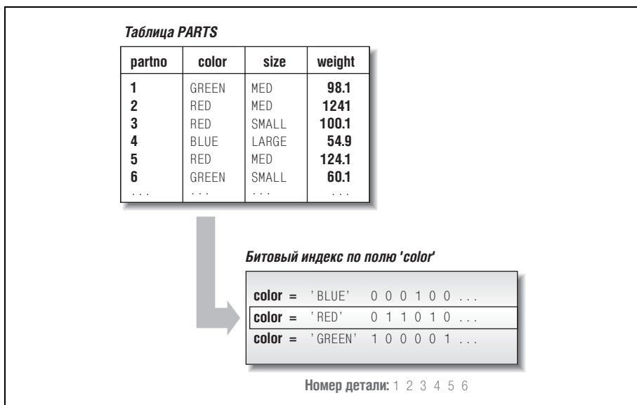
Рис. 4.2. Битовый индекс
