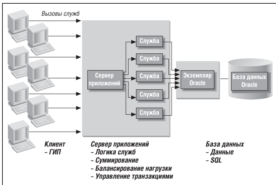
Рис. 9.3. Трехуровневая архитектура
