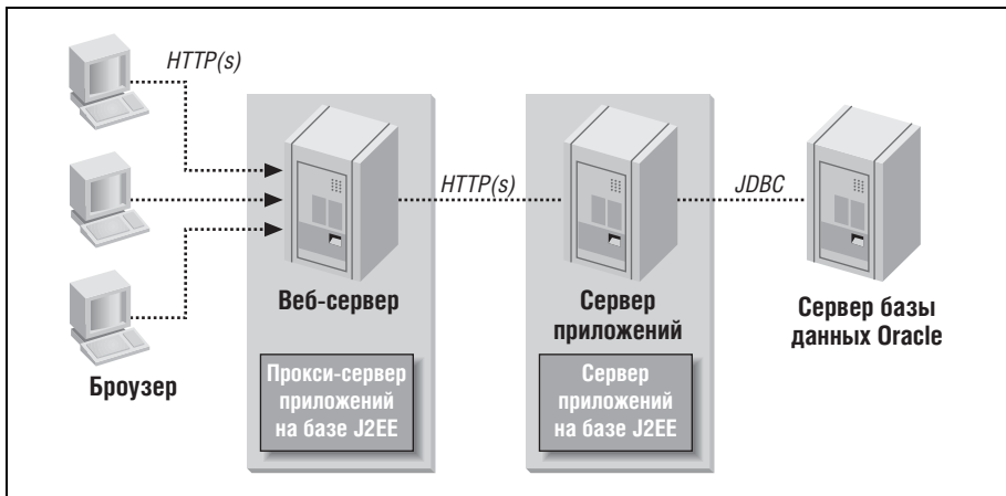
Рис. 9.4. N-уровневая система
