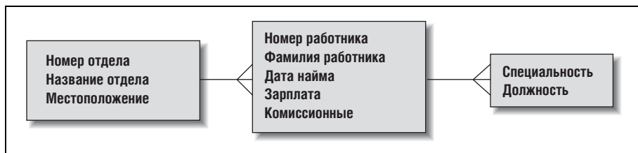
Рис. 4.3. Процедура нормализации
