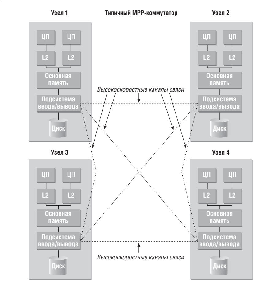
Рис.12.4. Массивно-параллельная система
