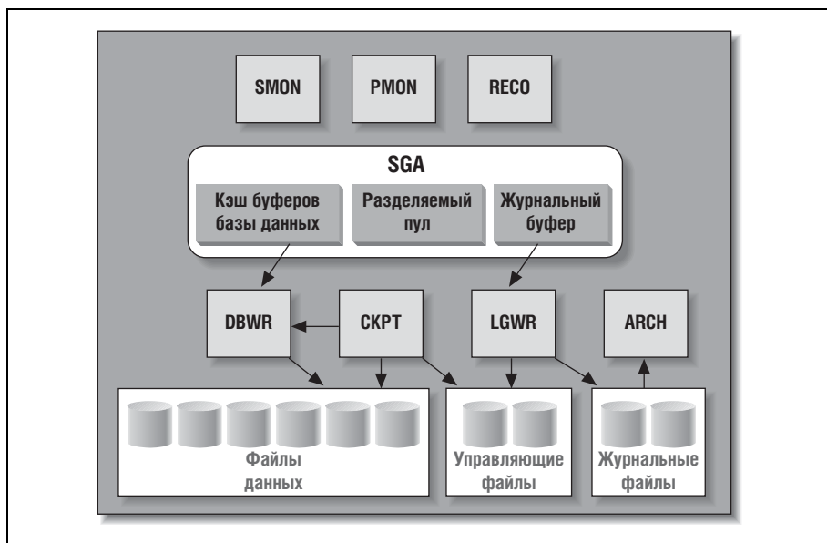
Рис. 2.8. Экземпляр Oracle
