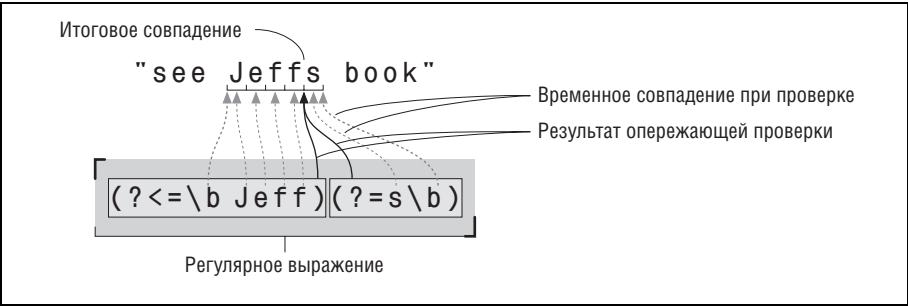
Рис. 2.7. Поиск совпадения для выражения (?<=\\b Jeff) (?=s\\b)
